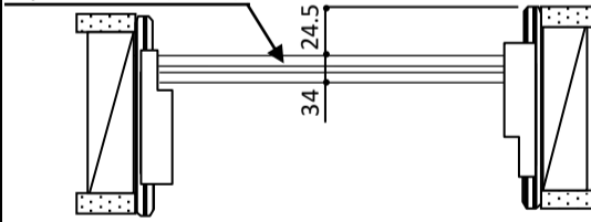
床付けレール(面付)は、所定位置にレール中央から両側に向かって付属ビスで取付
