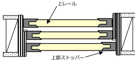
3枚引違い戸(非連動)・ソフトクローズ無しの場合に上部ストッパーを取付けます
