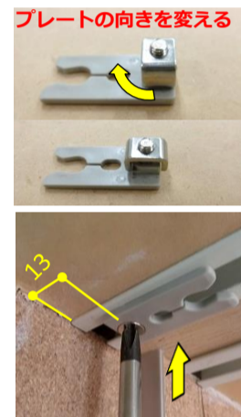
3枚引違い戸(非連動)・ソフトクローズ無しの場合に上部ストッパーを取付けます
