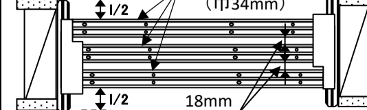
床付けレール(埋込V)は、所定位置に当て木をして、溝に埋め込む。
