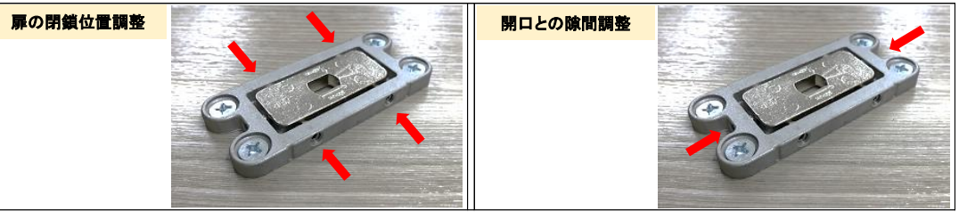
6箇所の調整ネジ（赤矢印部）を六角レンチ(M3)で 「扉の閉鎖位置」と「開口との隙間」を調整
