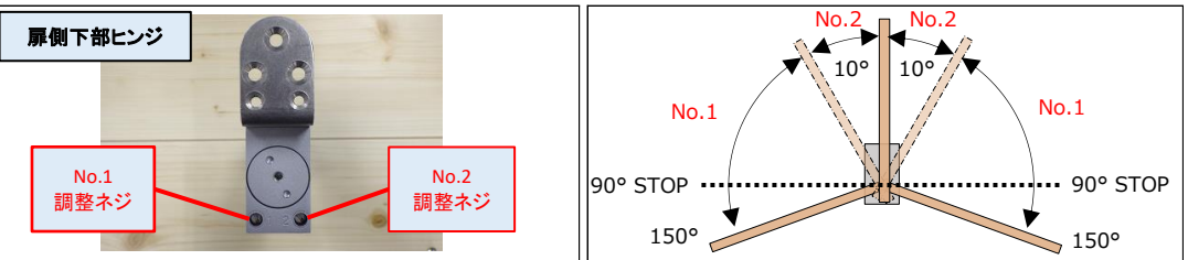
扉側の下部ヒンジにある開閉速度調整ネジ（No.1及びNo.2）を マイナスの手動ドライバーで回して開閉速度を調整
