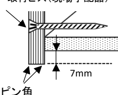
【クロス仕上の場合】 壁厚より7mmチリが出る
