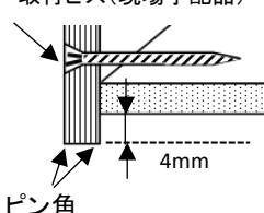
【塗り壁仕上の場合】 壁厚より4mmチリが出る
