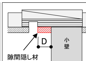
上枠下地のレール溝と小壁の間に 隙間隠し材を取りつける
