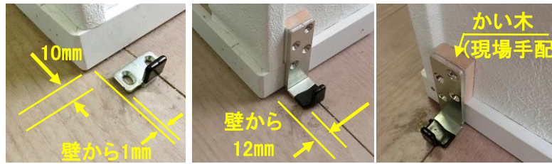
床付ガイドの場合
