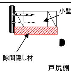
上枠下地のレール溝と小壁の間に 隙間隠し材を取りつける
