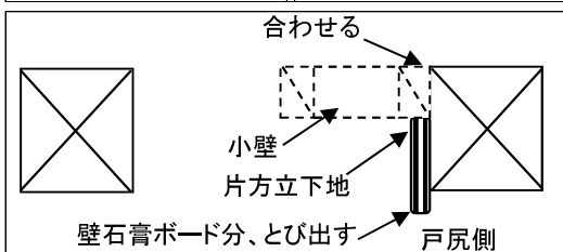
【片引き戸、2・3枚引込み戸】 片方立下地の取付位置
