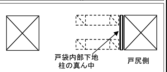
【ポケット戸】 戸袋内部下地の取付位置
