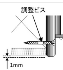
縦枠下地の見込寸法は壁厚+1mmずつのチリ
