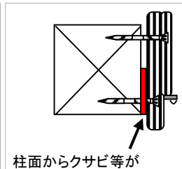
縦枠下地の下部裏側に2mm厚パッキン材取付済
