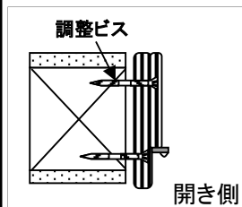
調整ビスにより枠を固定
