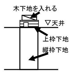
上枠下地の裏には木下地を入れる
