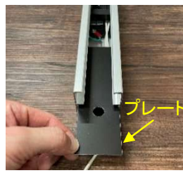
戸先側より プレートを抜く
