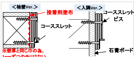
【準耐火納まりの場合】
