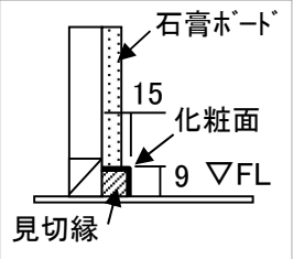
【準耐火納まりの場合】 入隅の場合は中方立下地は使用せず 石膏ボードを伸ばす
