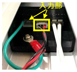
サブコードのコネクタを 入力部に差し込む ※入力部はどちら側でも 大丈夫です
