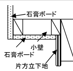
【準耐火納まりの場合】 入隅の場合は中方立下地は使用せず 石膏ボードを伸ばす
