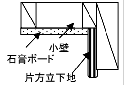
【準耐火納まりの場合】 入隅の場合は中方立下地は使用せず 石膏ボードを伸ばす
