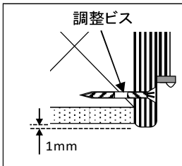
縦枠下地の見込寸法は壁厚+1mmずつのチリ
