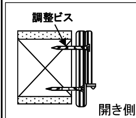
調整ビスにより枠を固定
