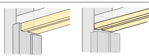
【縦枠勝ち】 → 【上枠勝ち】
